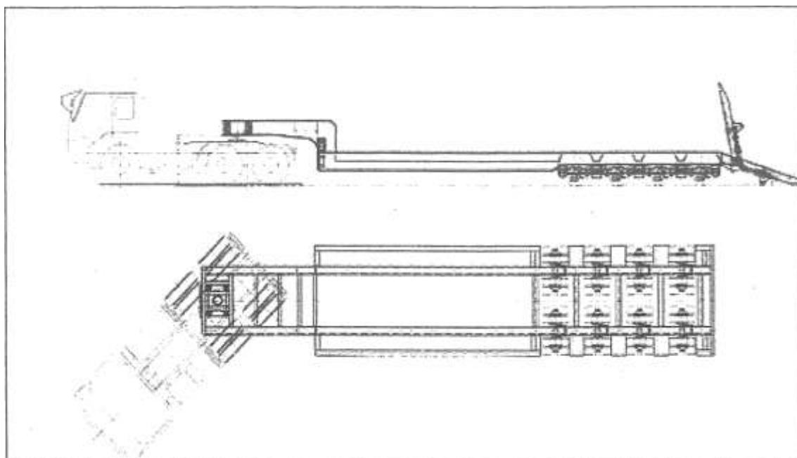
Skema teknike tërheqës plus gjysëmrimorkio
