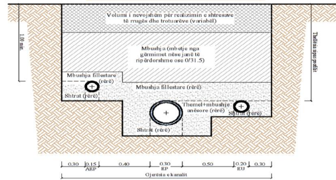
Kanal për rrjetin e furnizimit me ujë të pijshëm, ujrë e zeza dhe ujërë të shiut
