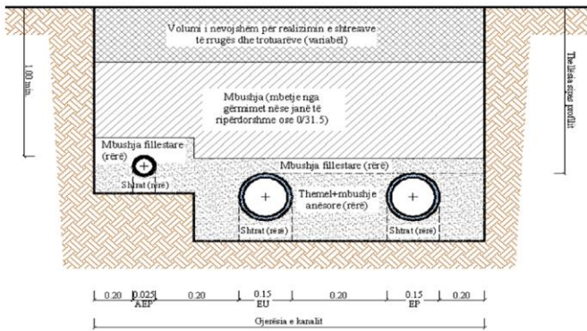
Kanal për rrjetin e gazit, telekomit, UPC, elektrikut dhe të ndriçimit të rrugëve
