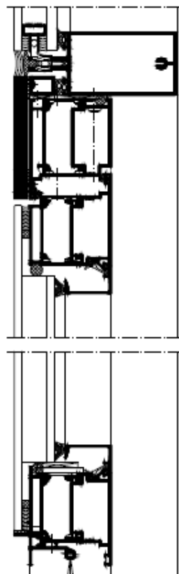
⑫ Naßversiegelung Wet sealing
