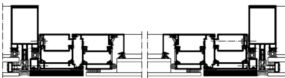
⑬ Naßversiegelung Wet sealing
